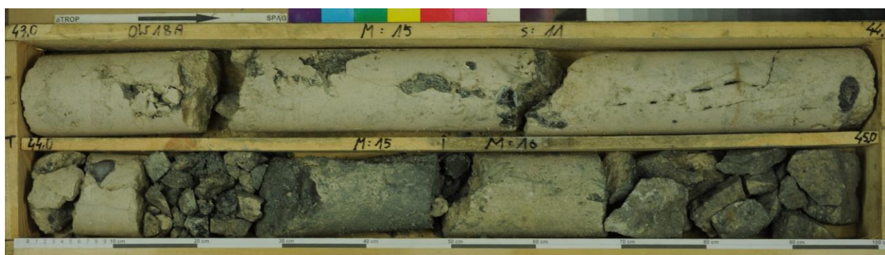
Fotografia 3 Zdjęcie rdzenia z wiercenia OW-18a (rejon Plant Krakowskich) ukazujące warstwę wapieni jurajskich z głębokości 43-45m p.p.t.
