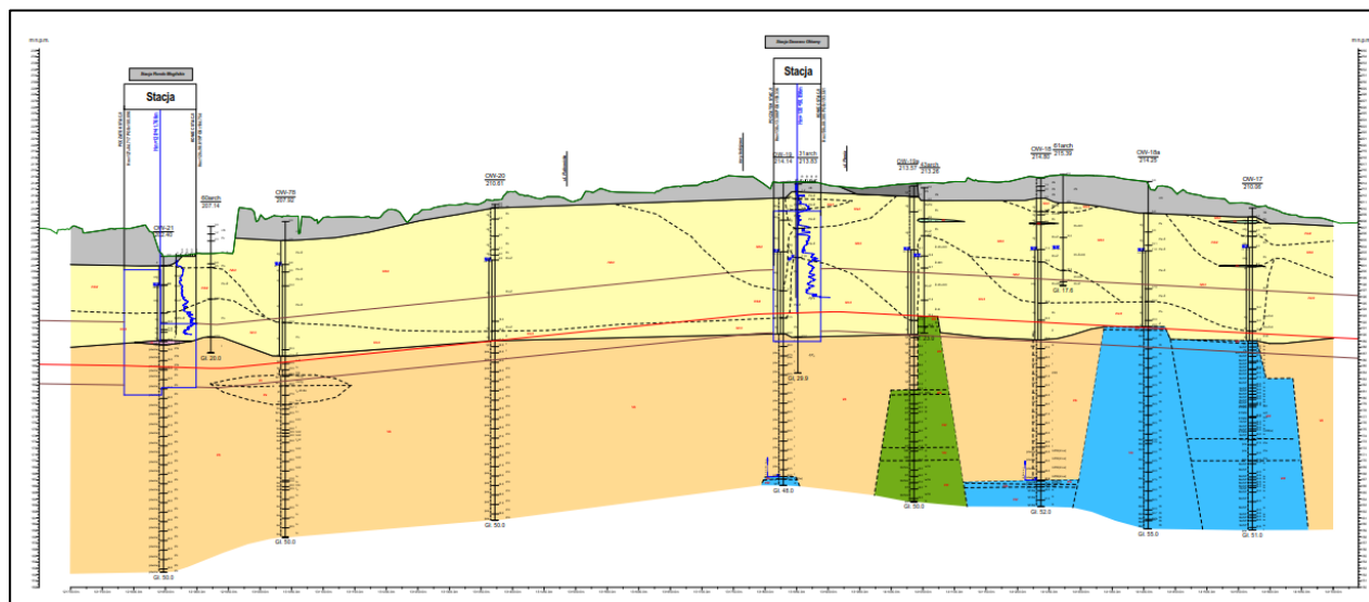
Rysunek 24 Przykładowy przekrój w obrębie odcinka od stacji Rondo Mogiłskie – Dworzec Główny – odcinek tunelowy do stacji Stare Miasto dla wariantu T6D tramwaju ukazujący lokalizację wychodni utworów starszych (jurajsko - kredowych).
