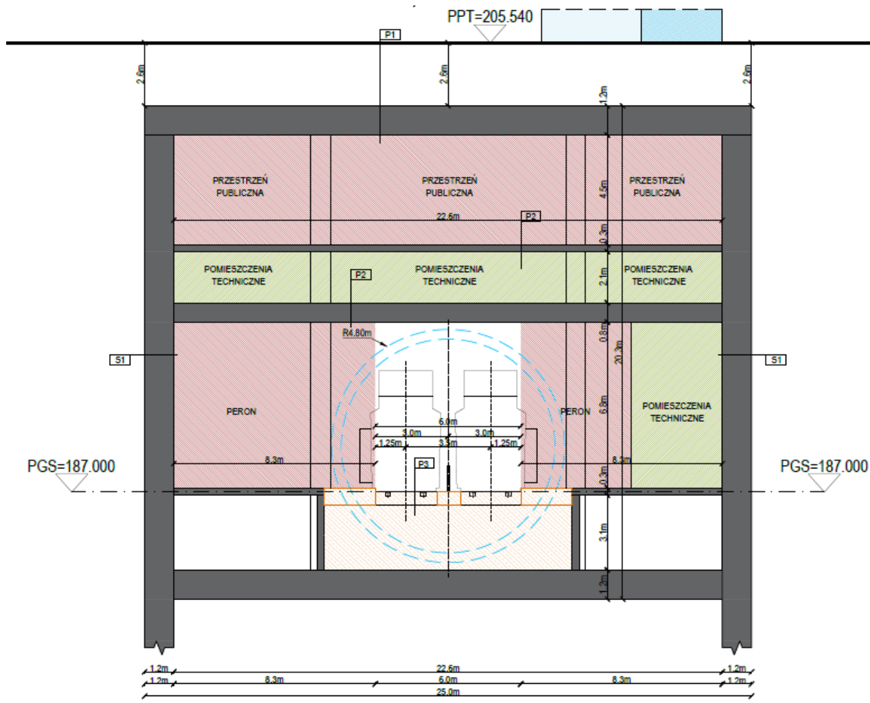
Rysunek 19 Przykładowy przekrój poprzeczny dla przystanku podziemnego premetra szybkiego tramwaju
