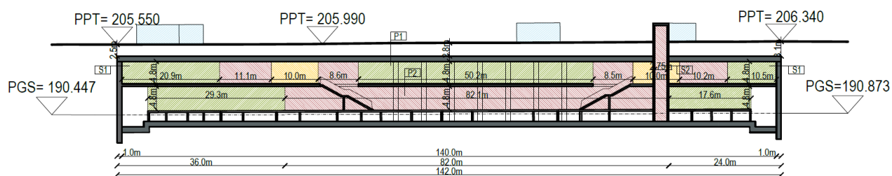
Rysunek 20 Przykładowy przekrój podłużny stacji metra
