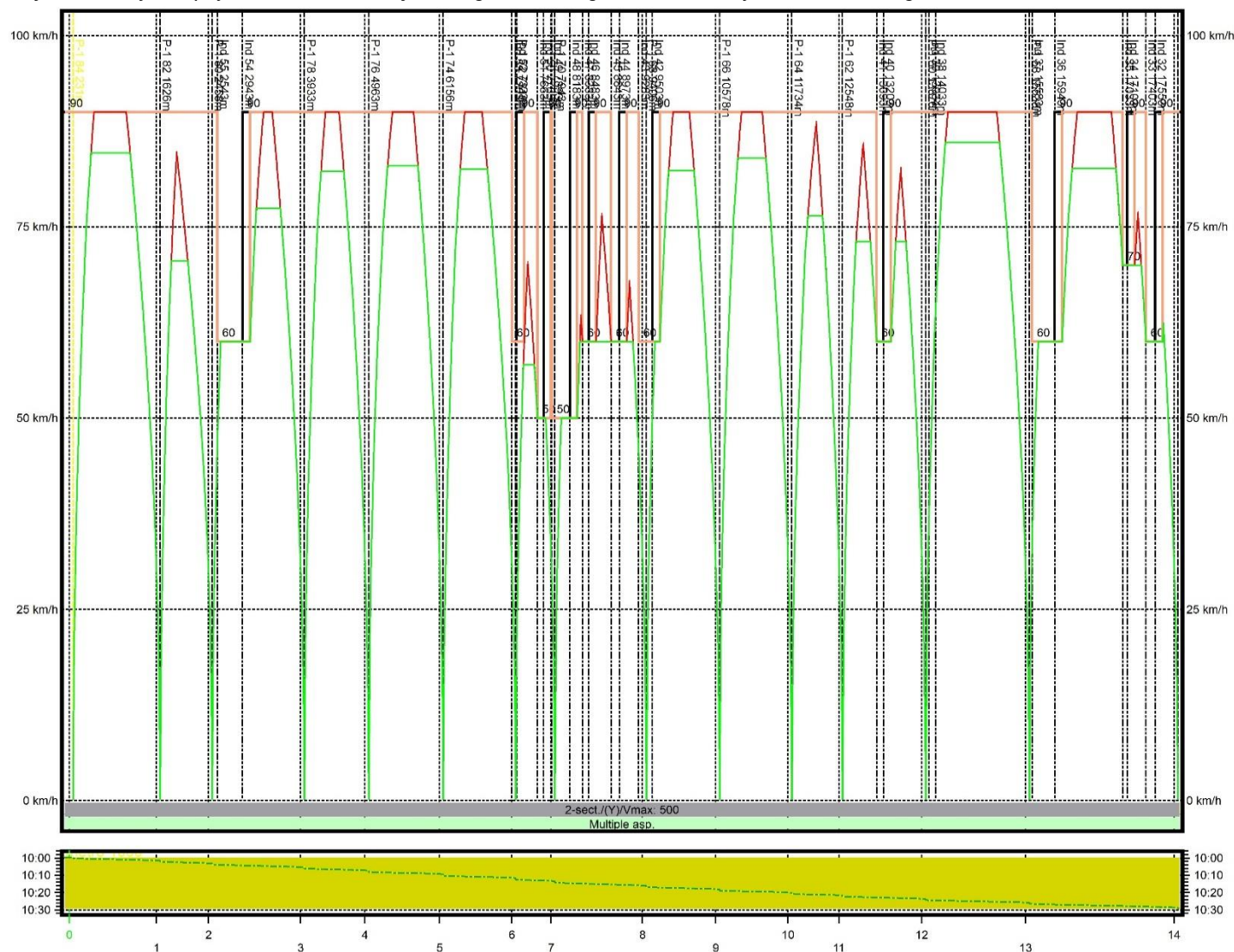
Wykres 19 Wykres prędkości W4d w relacji Jasnogórska – Mogiła, W4c w relacji Bronowice - Mogiła
