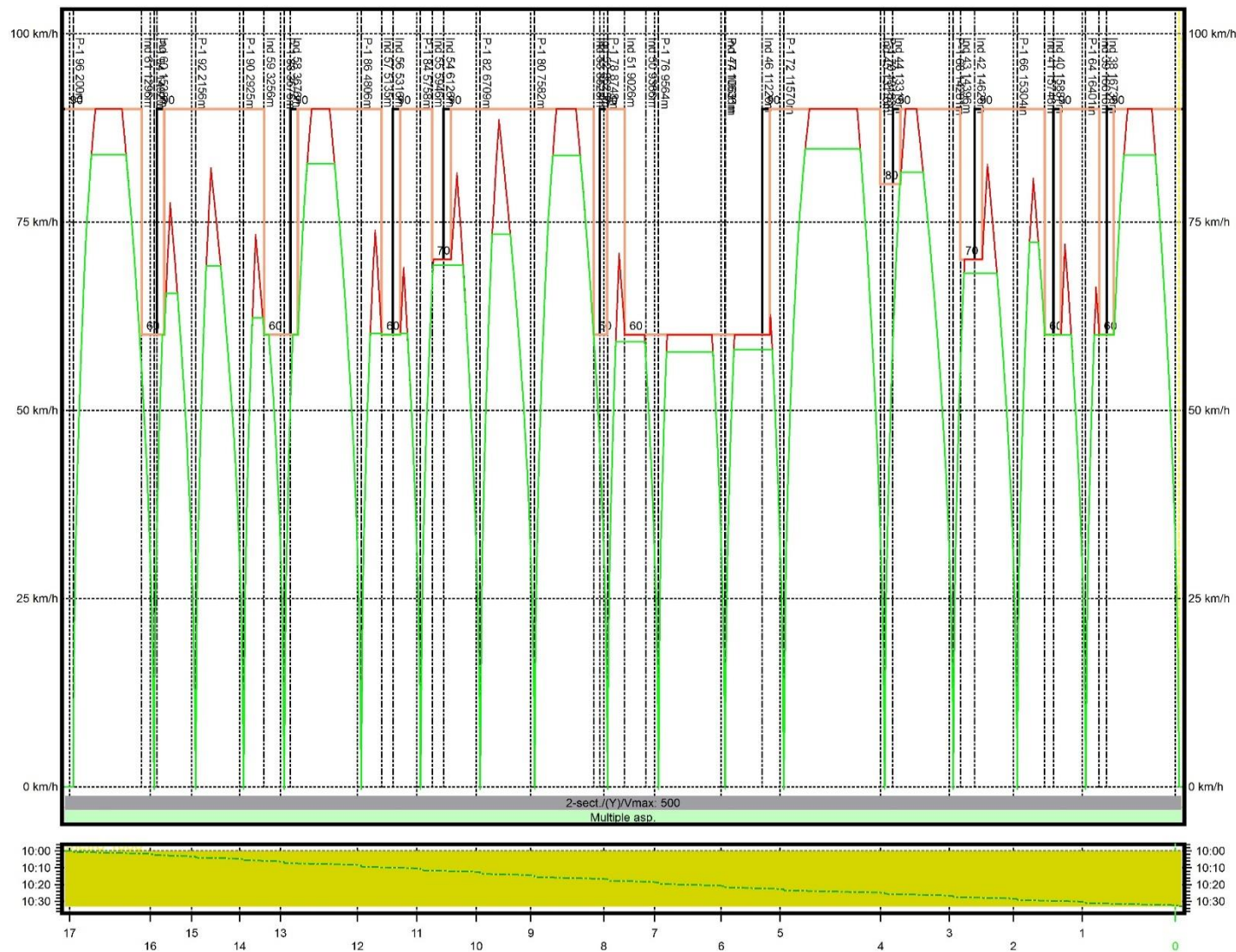
Wykres 23 Wykres prędkości W5b w relacji Jasnogórska - Kombinat
