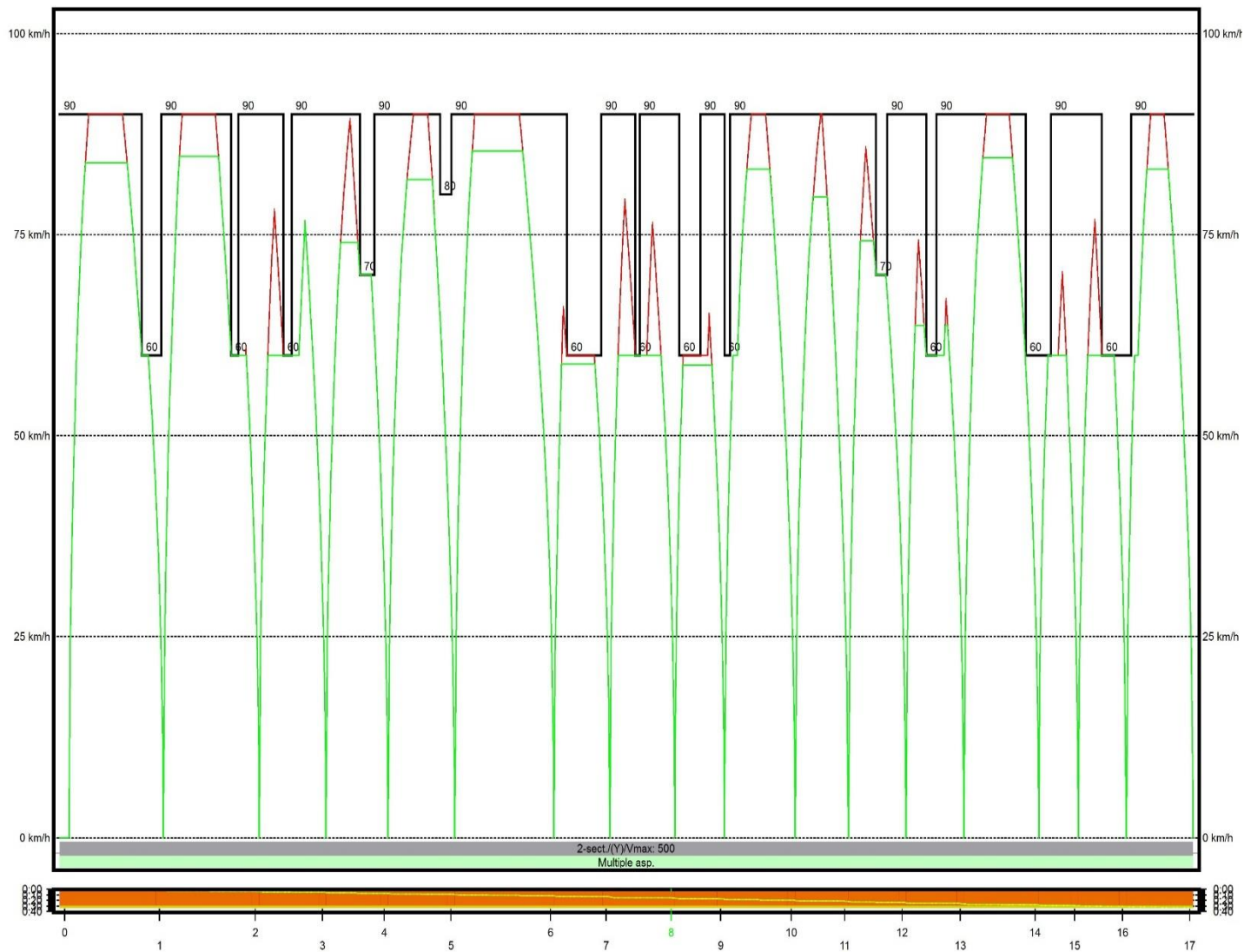
Wykres 26 Wykres prędkości W5c w relacji Wzgórza Krzesławickie - Bronowice
