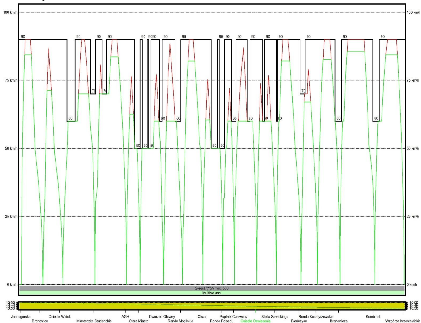
Wykres 29 Wykres prędkości W6d w relacji Jasnogórska - Wzgórza Krzesławickie, W6a Bronowice – Kombinat, W6b Jasnogórska – Kombinat, W6d Bronowice – Wzgórza Krzesławickie
