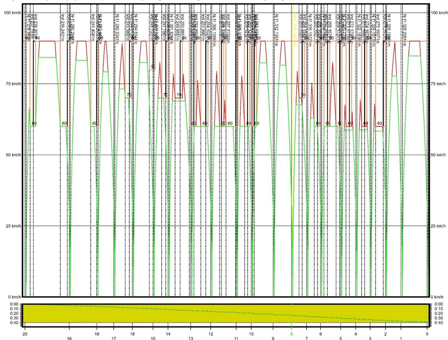
Wykres 4 Wykres prędkości W1b w relacji Mogiła - Jasnogórska, W1d w relacji Mogiła - Bronowice
