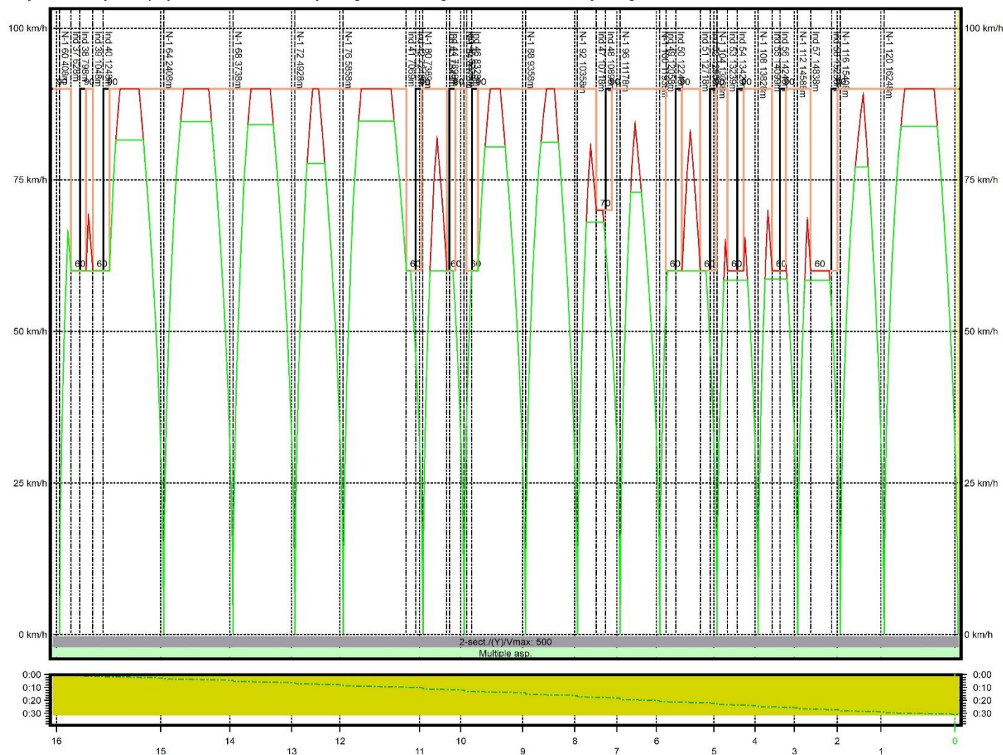
Wykres 6 Wykres prędkości W2c w relacji Mogiła - Jasnogórska, W2a w relacji Mogiła - Bronowice
