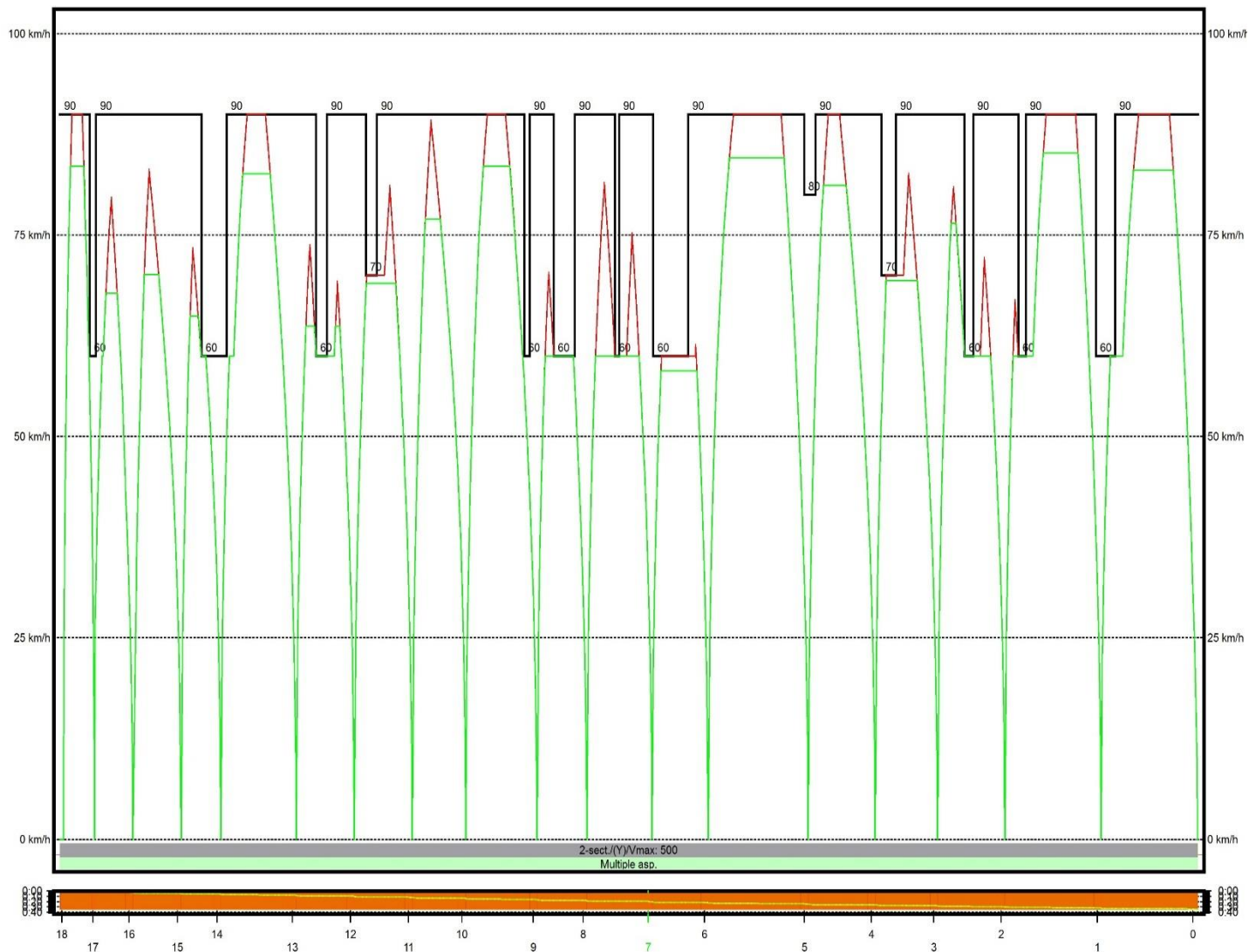
Wykres 28 Wykres prędkości W5d w relacji Jasnogórska - Wzgórza Krzesławickie
