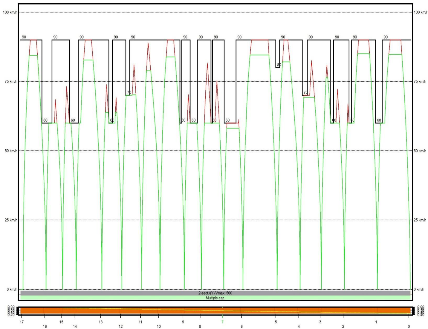
Wykres 25 Wykres prędkości W5c w relacji Bronowice – Wzgórza Krzesławickie
