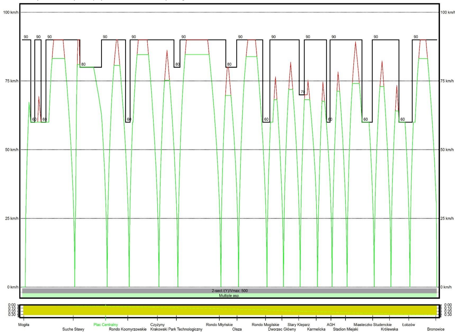
Wykres 10 Wykres prędkości W3a w relacji Mogiła – Bronowice
