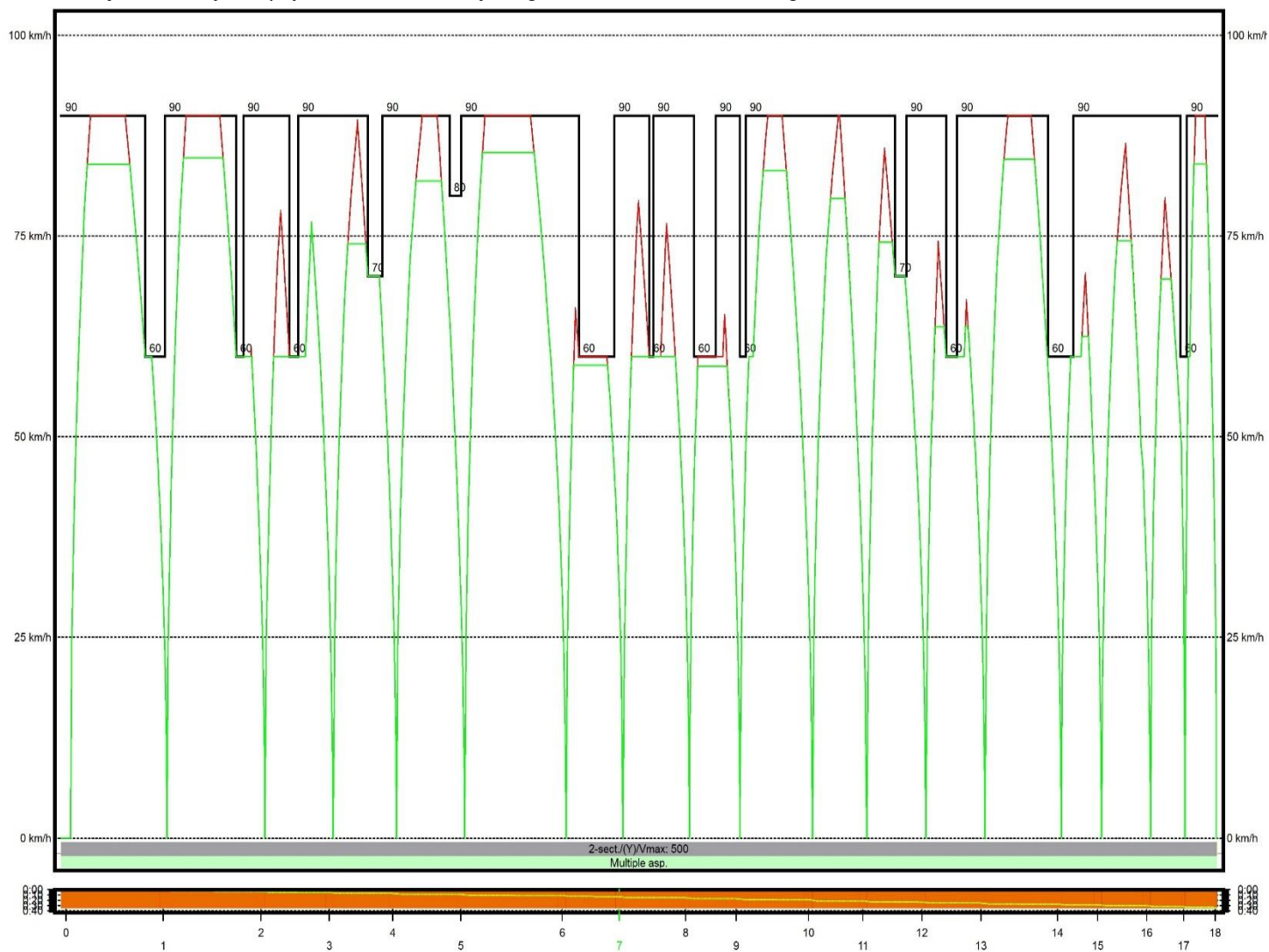
Wykres 27 Wykres prędkości W5d w relacji Wzgórza Krzesławickie - Jasnogórska
