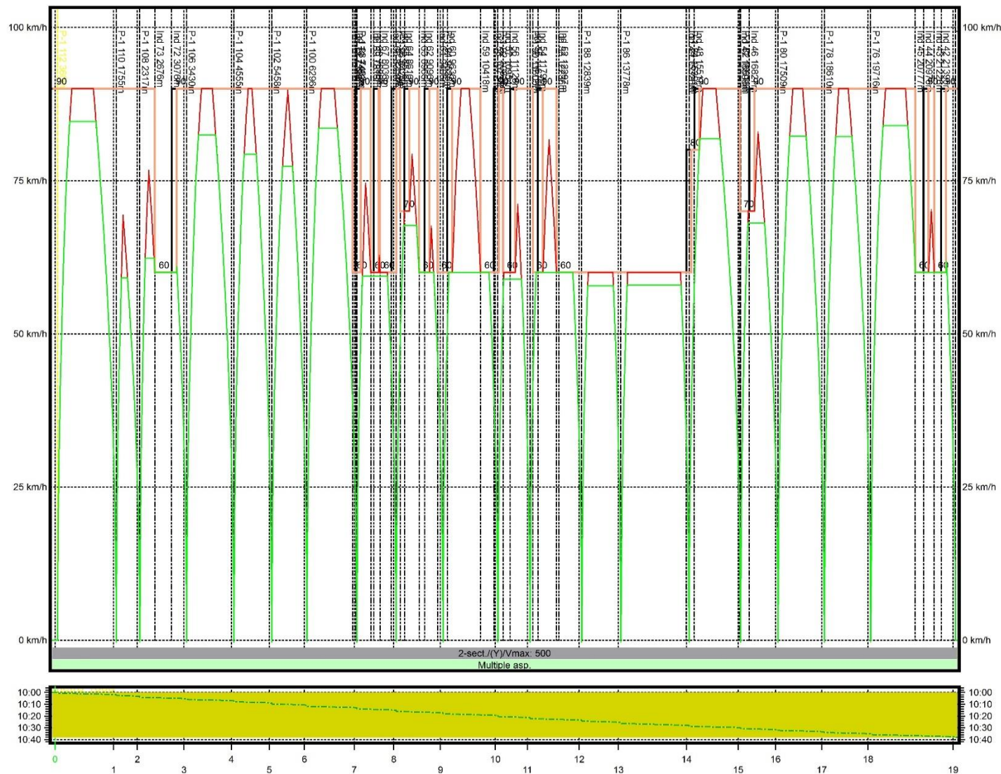
Wykres 31 Wykres prędkości W7c w relacji Jasnogórska – Mogiła, W7a w relacji Bronowice – Mogiła
