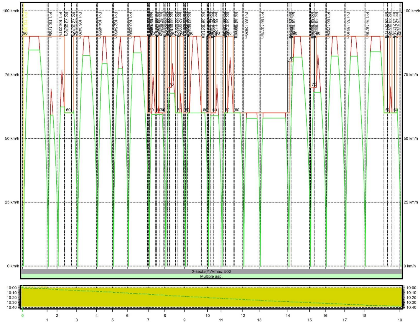
Wykres 32 Wykres prędkości W7c w relacji Mogiła - Jasnogórska, W7a w relacji Mogiła - Bronowice
