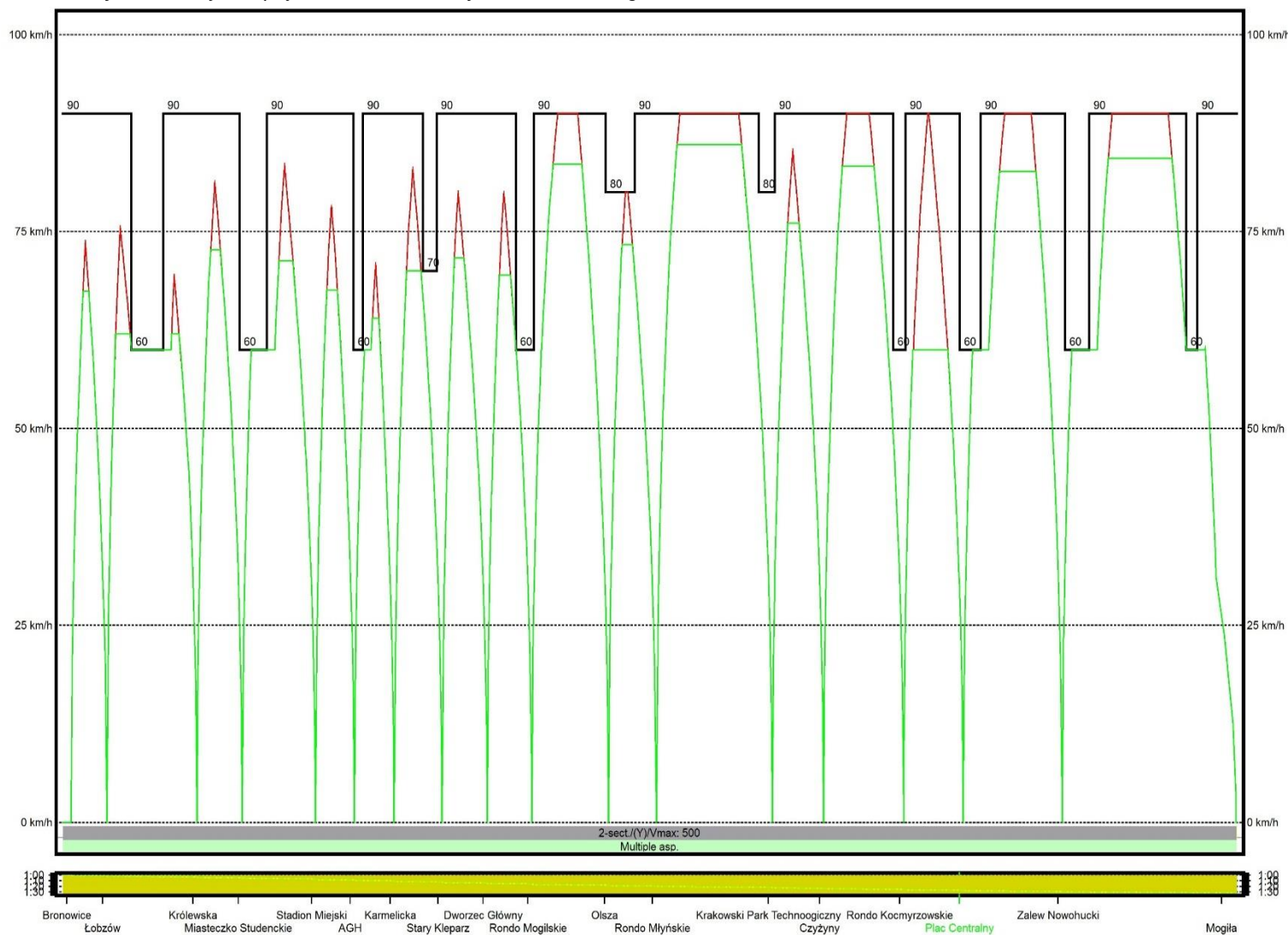
Wykres 13 Wykres prędkości W3c w relacji Bronowice - Mogiła
