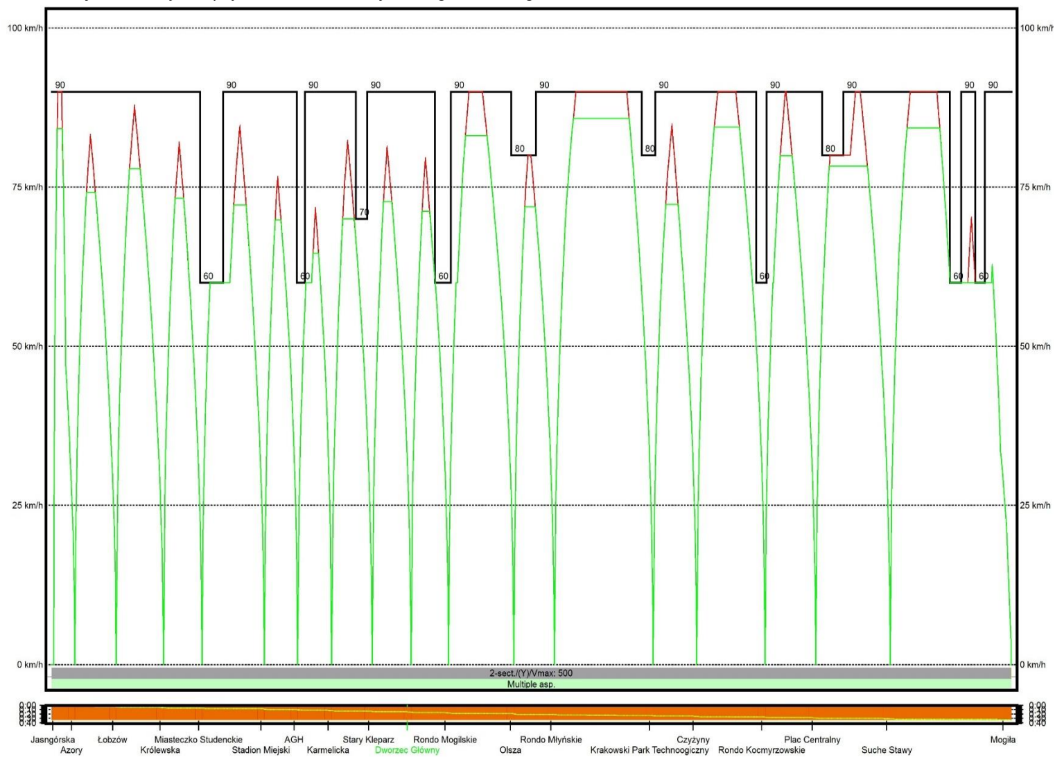
Wykres 11 Wykres prędkości W3b w relacji Jasnogórska - Mogiła
