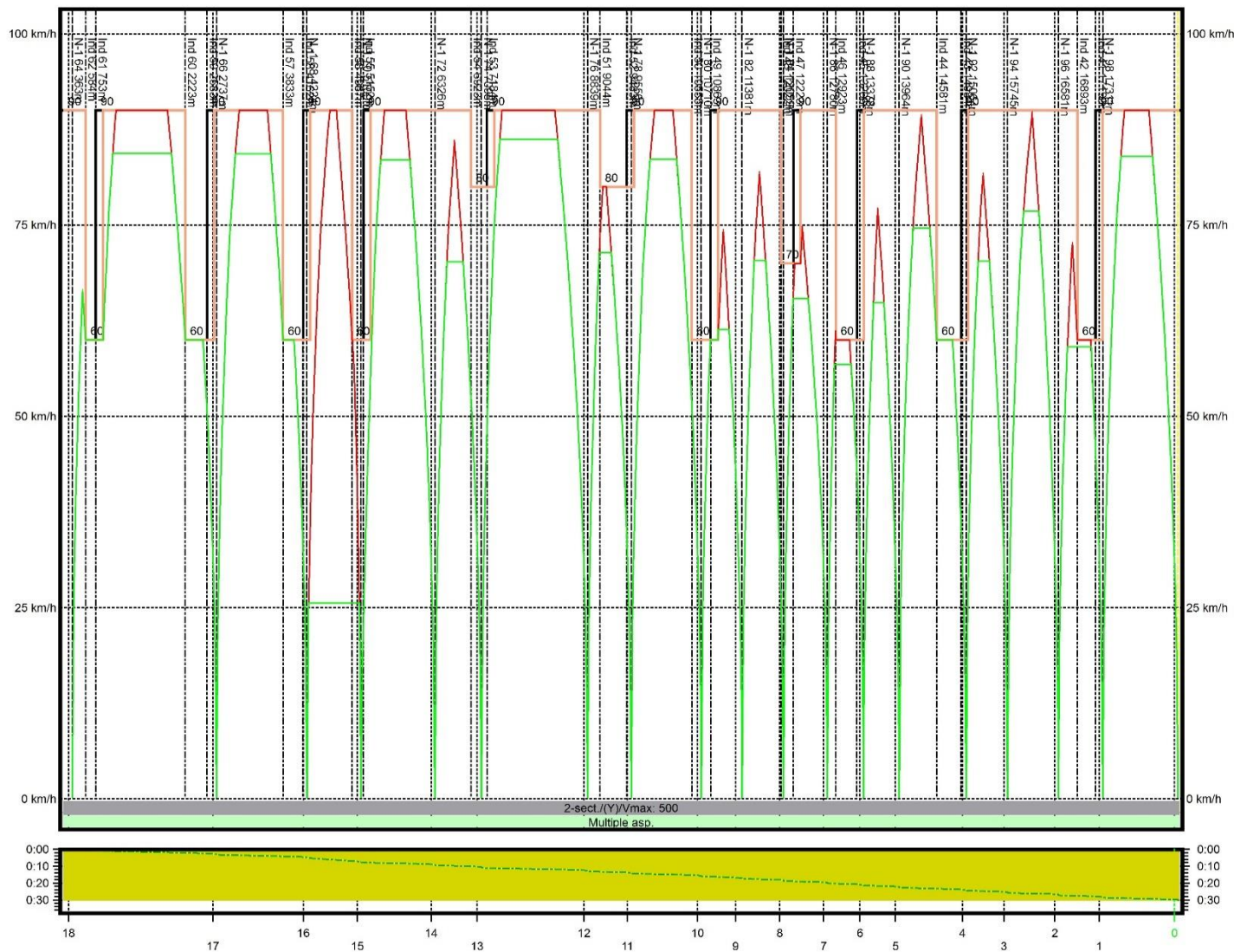
Wykres 16 Wykres prędkości W3d w relacji Mogiła - Jasnogórska
