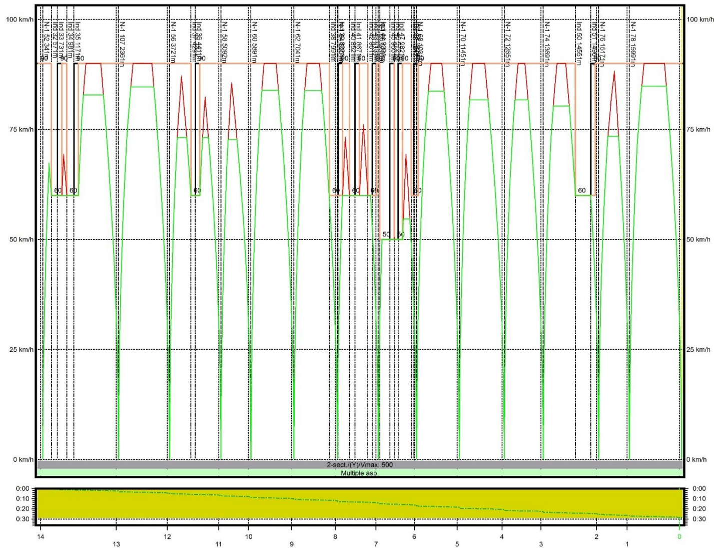
Wykres 18 Wykres prędkości W4b w relacji Mogiła - Jasnogórska, W4a w relacji Mogiła - Bronowice
