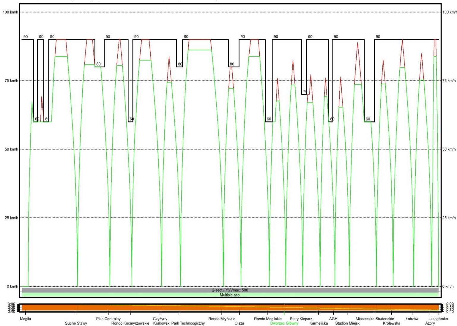
Wykres 12 Wykres prędkości W3b w relacji Mogiła - Jasnogórska
