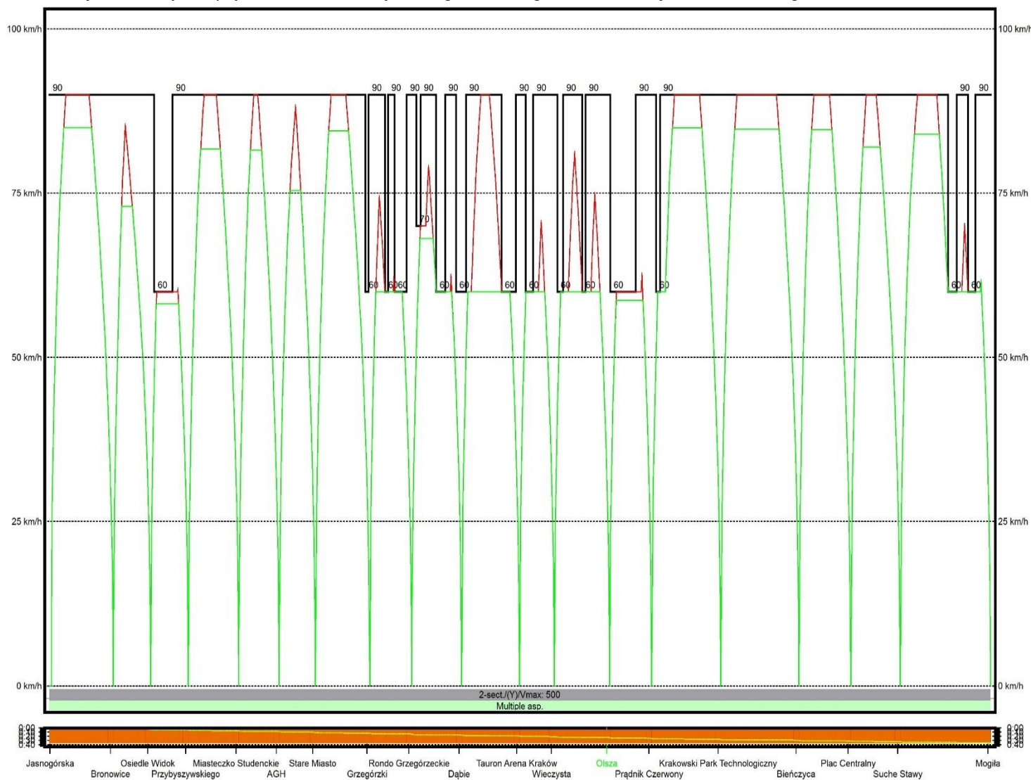
Wykres 34 Wykres prędkości W7d w relacji Jasnogórska - Mogiła, W7b w relacji Bronowice - Mogiła
