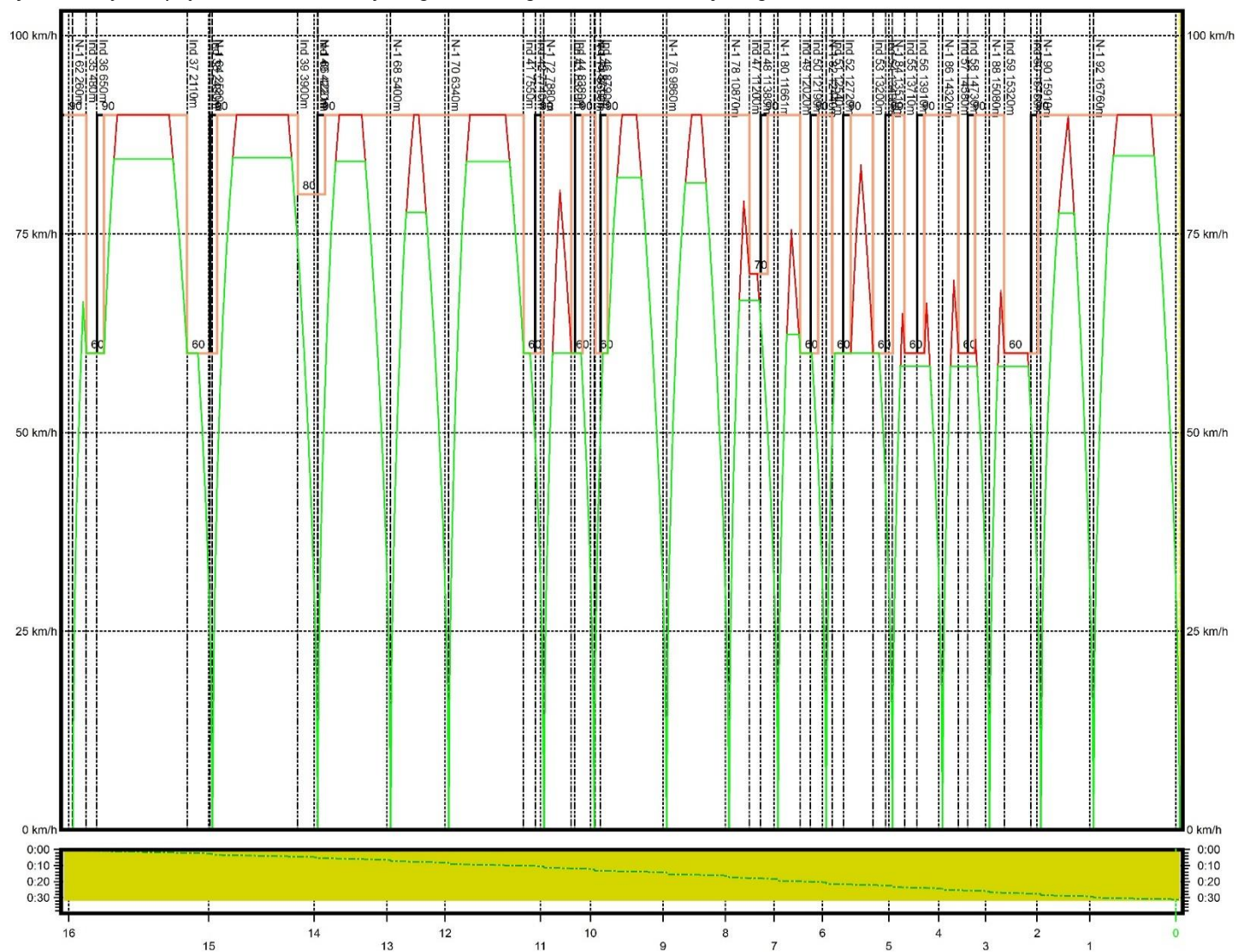
Wykres 8 Wykres prędkości W2d w relacji Mogiła - Jasnogórska, W2b w relacji Mogiła - Bronowice
