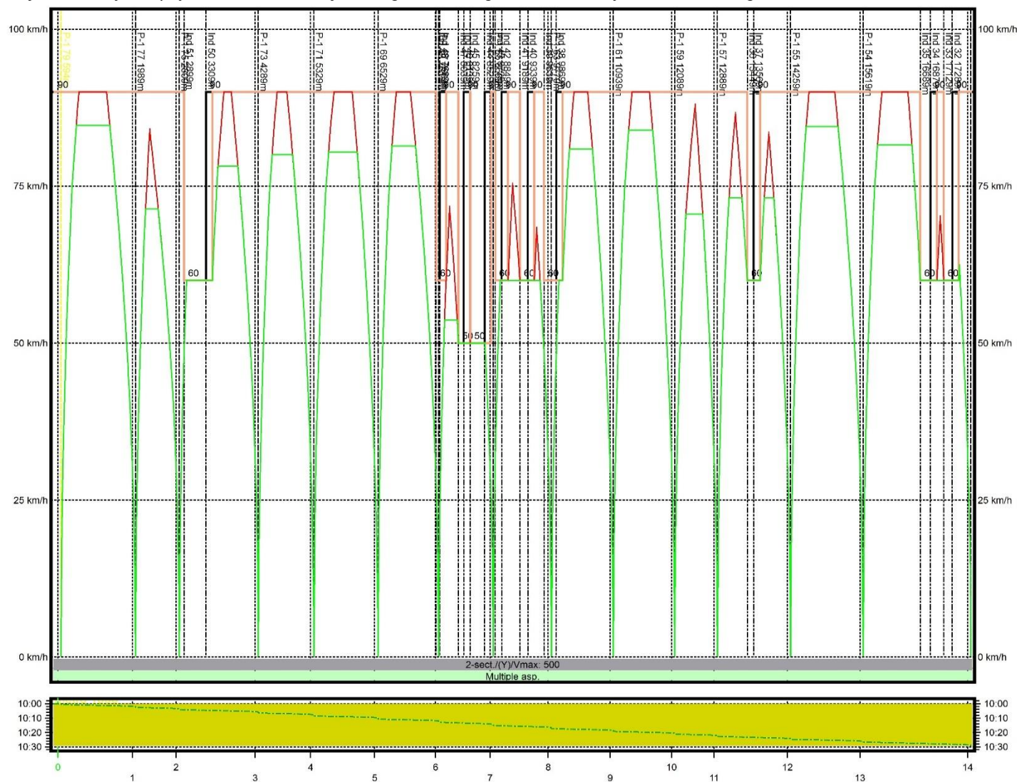
Wykres 17 Wykres prędkości W4b w relacji Jasnogórska – Mogiła, W4a w relacji Bronowice - Mogiła
