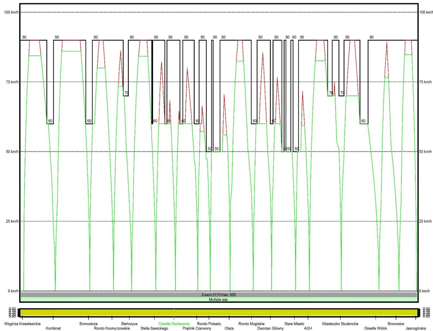
Wykres 30 Wykres prędkości W6d w relacji Wzgórza Krzesławickie - Jasnogórska, W6a Kombinat - Bronowice, W6b Kombinat - Jasnogórska, W6d Wzgórza Krzesławickie - Bronowice
