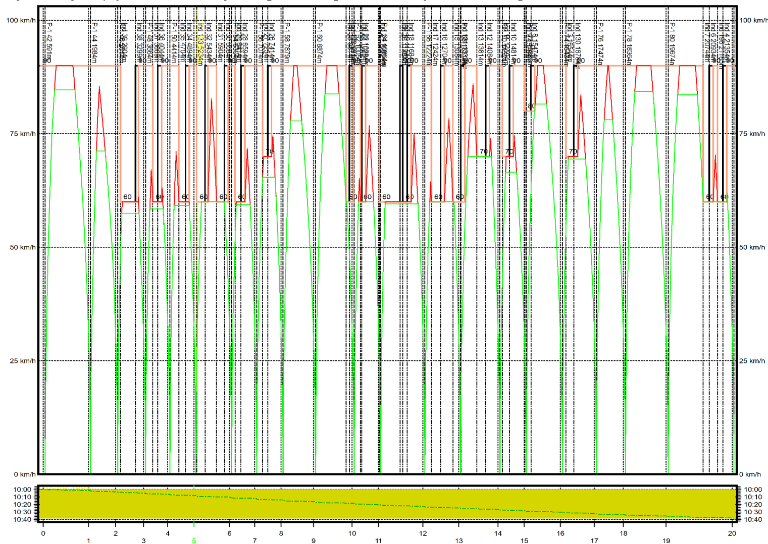
Wykres 1 Wykres prędkości W1a w relacji Jasnogórska – Mogiła, W1c w relacji Bronowice - Mogiła
