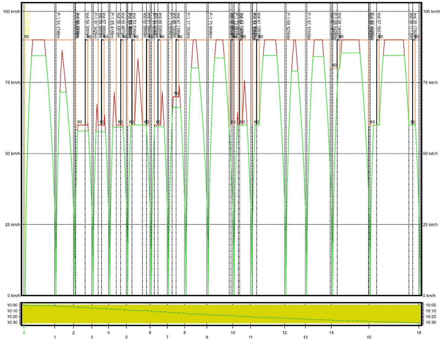
Wykres 7 Wykres prędkości W2d w relacji Jasnogórska – Mogiła, W2b w relacji Bronowice - Mogiła
