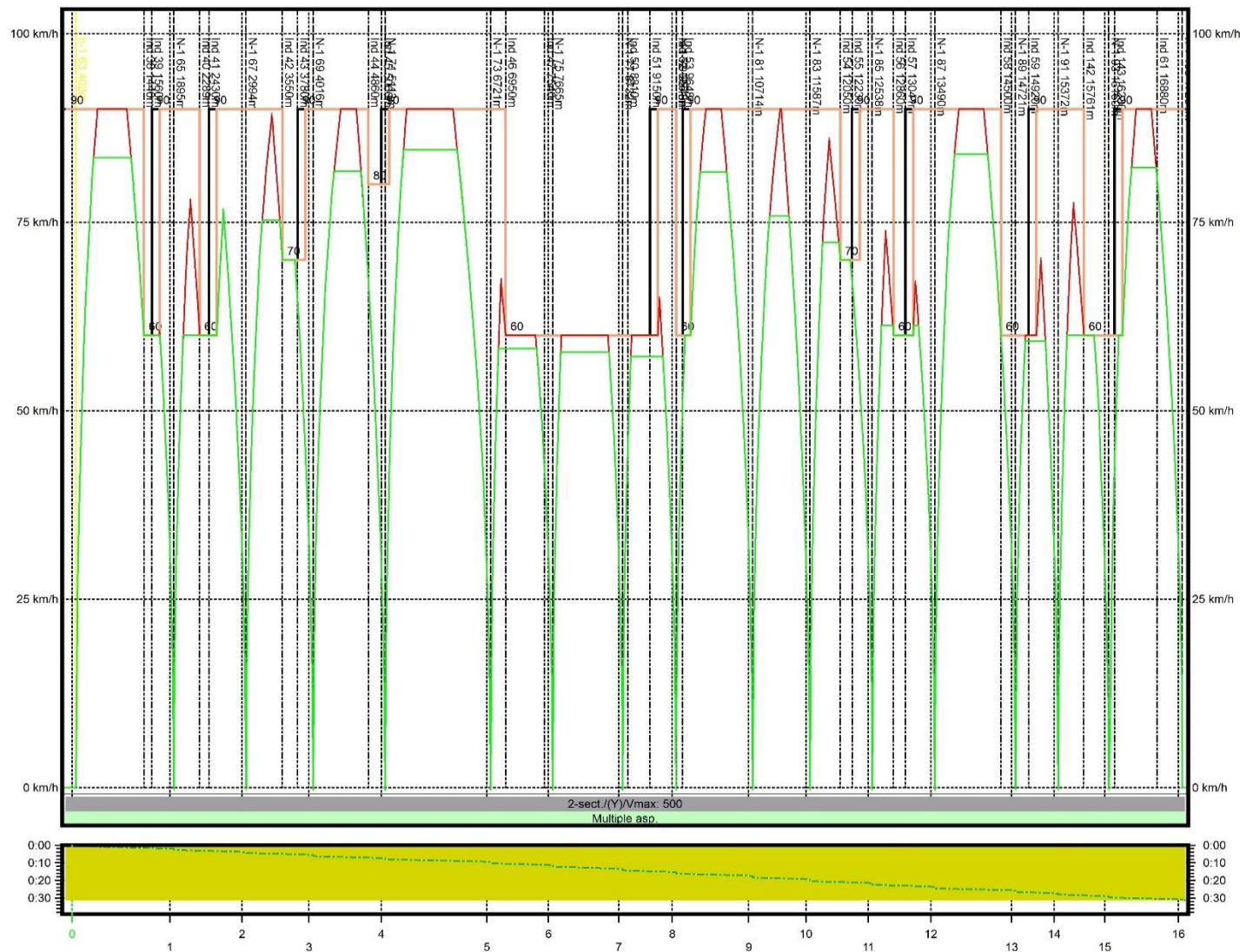
Wykres 21 Wykres prędkości W5a w relacji Kombinat - Bronowice
