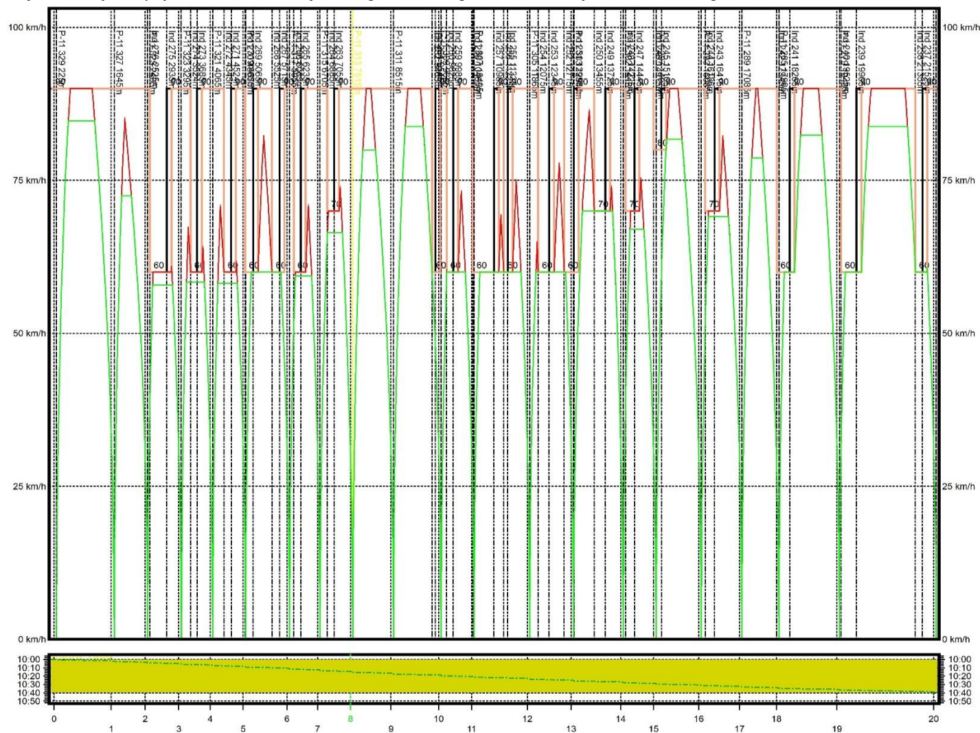
Wykres 3 Wykres prędkości W1b w relacji Jasnogórska – Mogiła, W1d w relacji Bronowice - Mogiła
