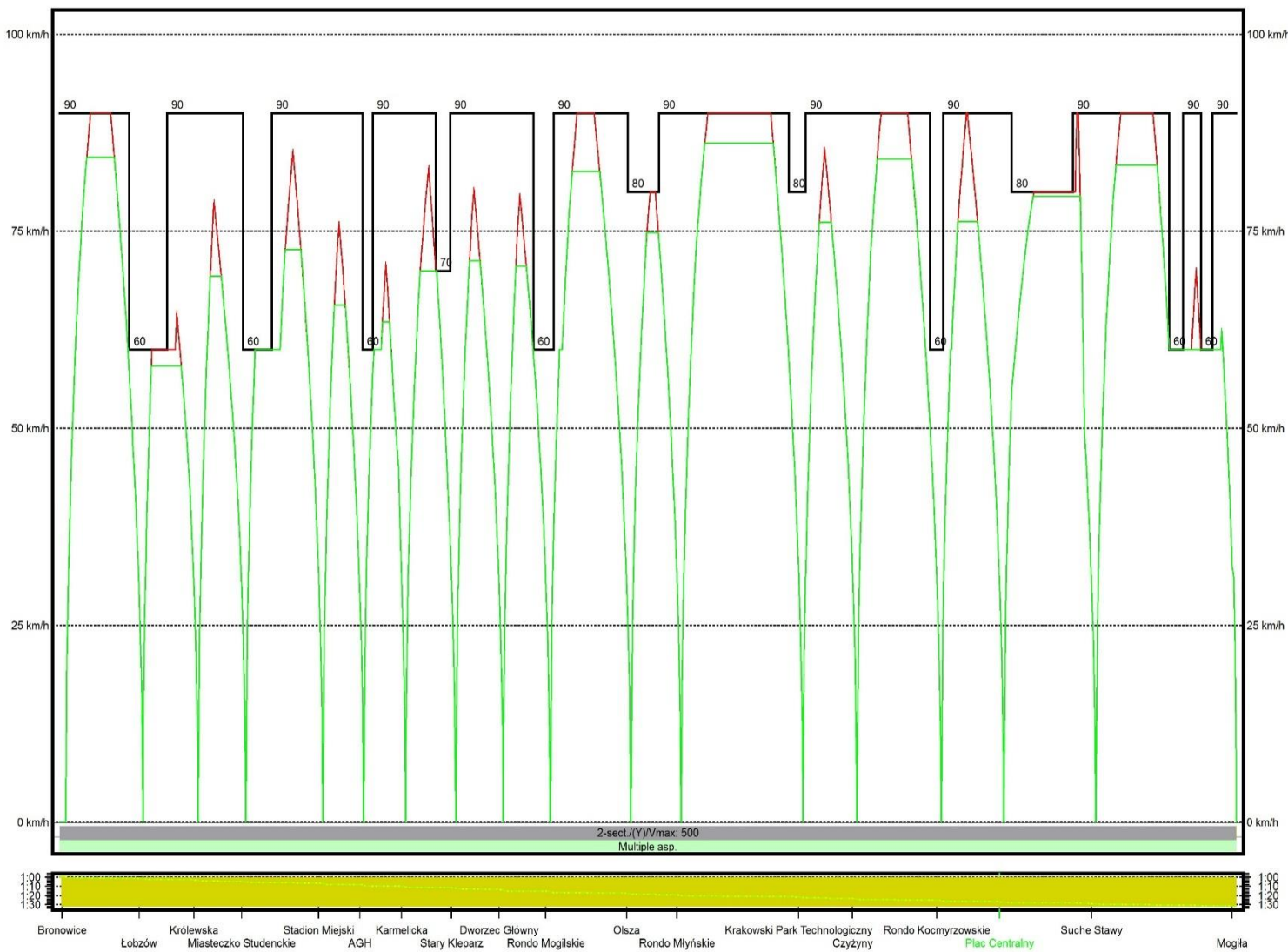
Wykres 9 Wykres prędkości W3a w relacji Bronowice – Mogiła
