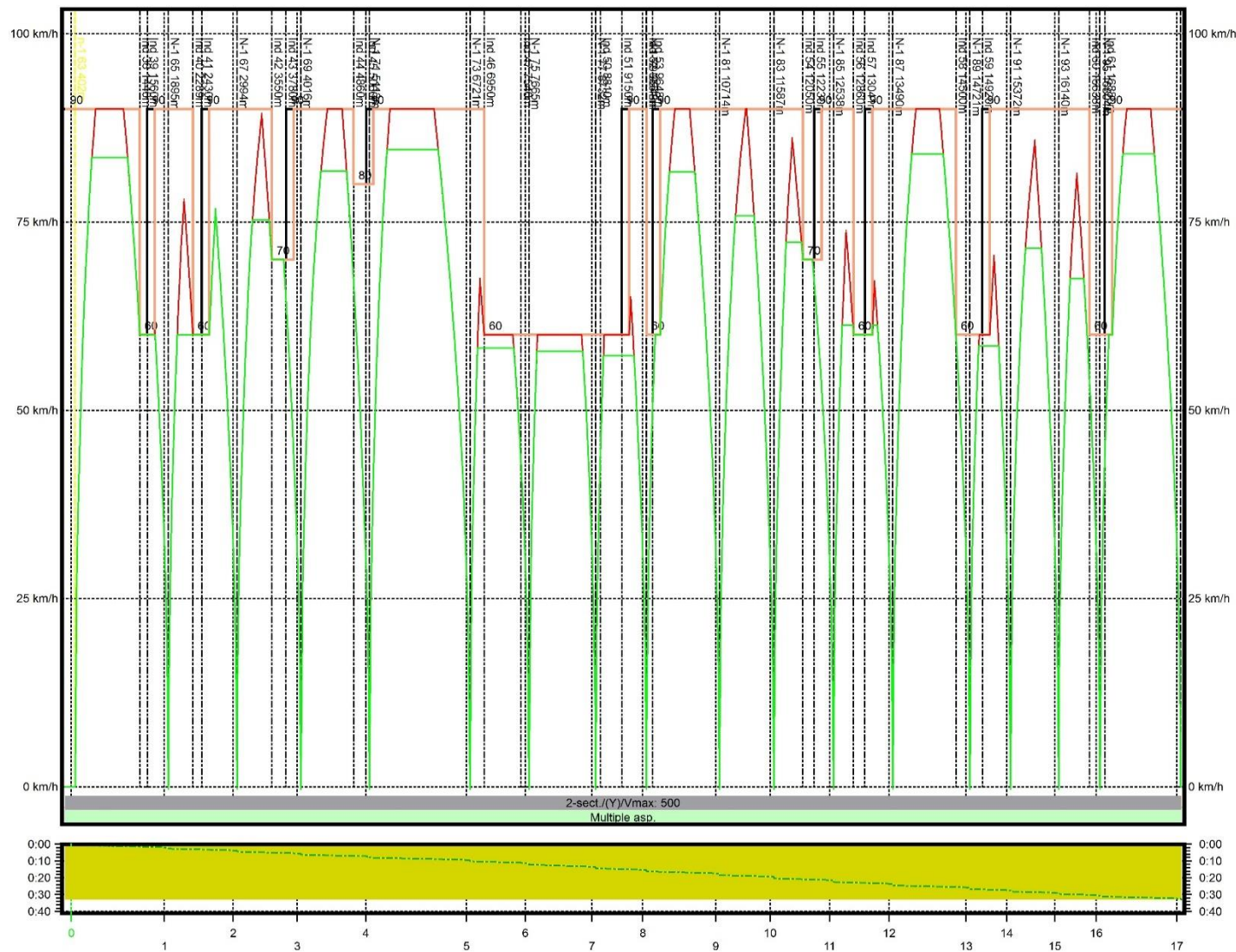
Wykres 24 Wykres prędkości W5b w relacji Kombinat - Jasnogórska
