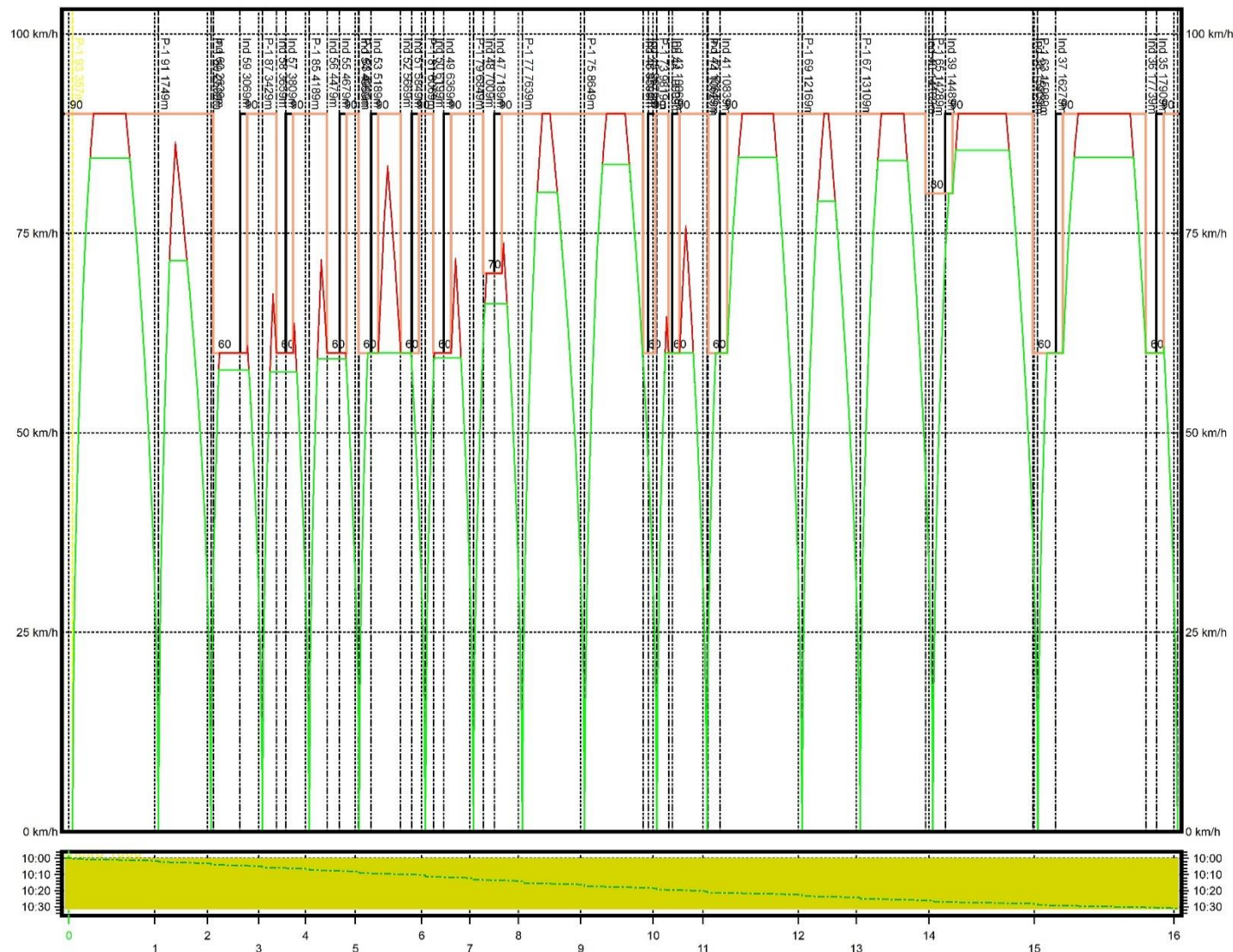
Wykres 15 Wykres prędkości W3d w relacji Jasnogórska – Mogiła
