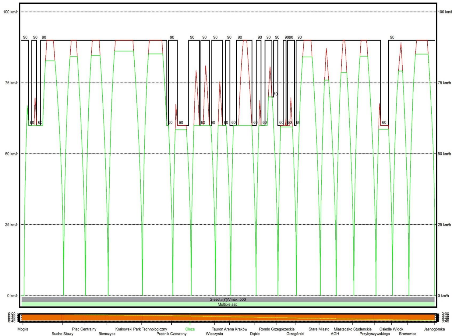
Wykres 33 Wykres prędkości W7d w relacji Mogiła - Jasnogórska, W7b w relacji Mogiła - Bronowice
