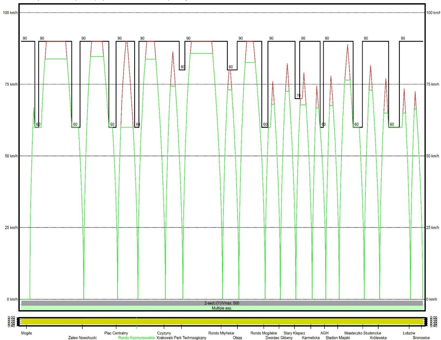
Wykres 14 Wykres prędkości W3c w relacji Mogiła - Bronowice
