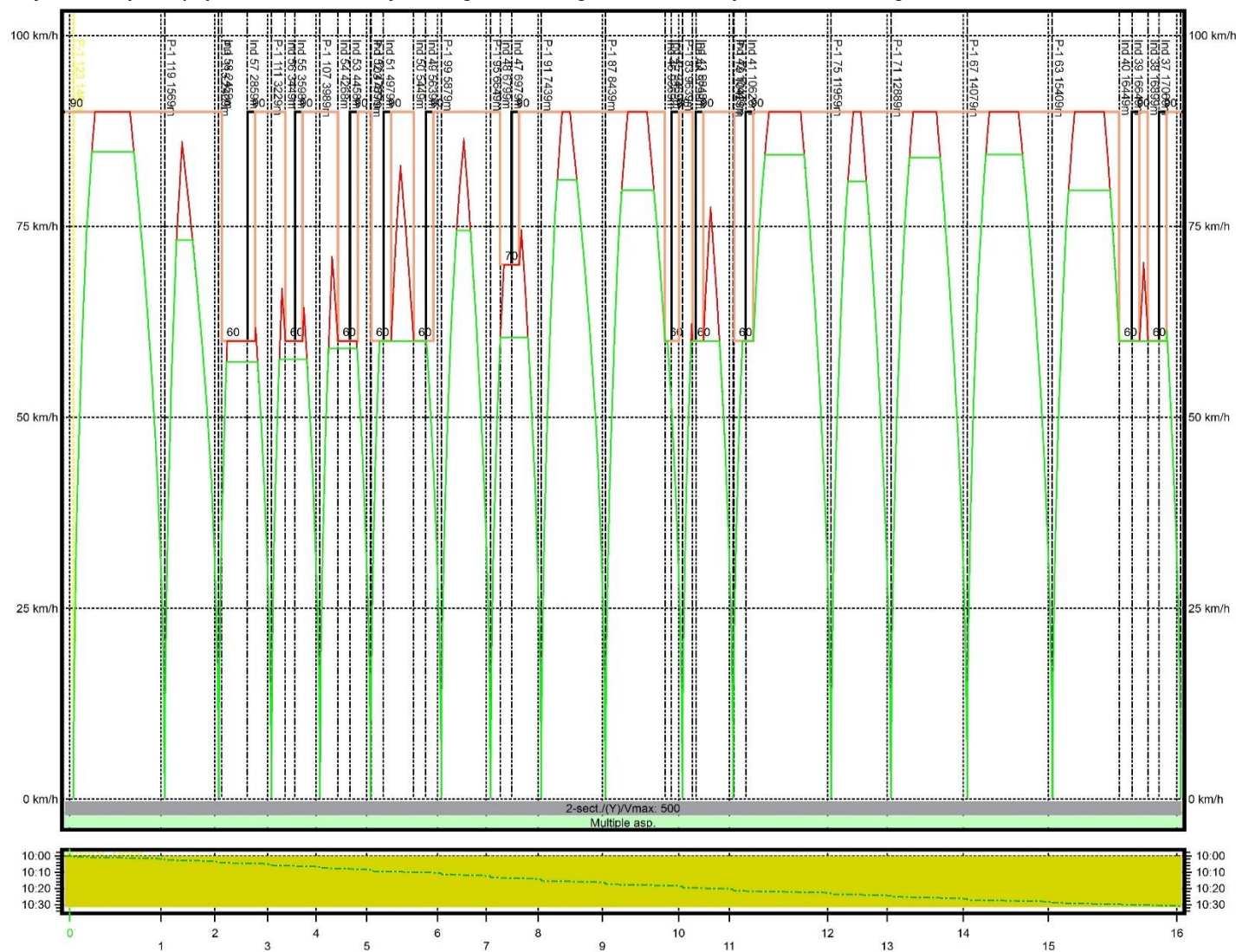
Wykres 5 Wykres prędkości W2c w relacji Jasnogórska – Mogiła, W2a w relacji Bronowice - Mogiła
